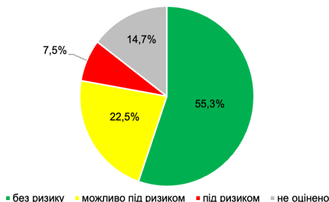
Рисунок 9. Оцінка ризику досягнення доброго екологічного стану / потенціалу за результатами оцінки антропогенних навантажень від дифузних джерел
