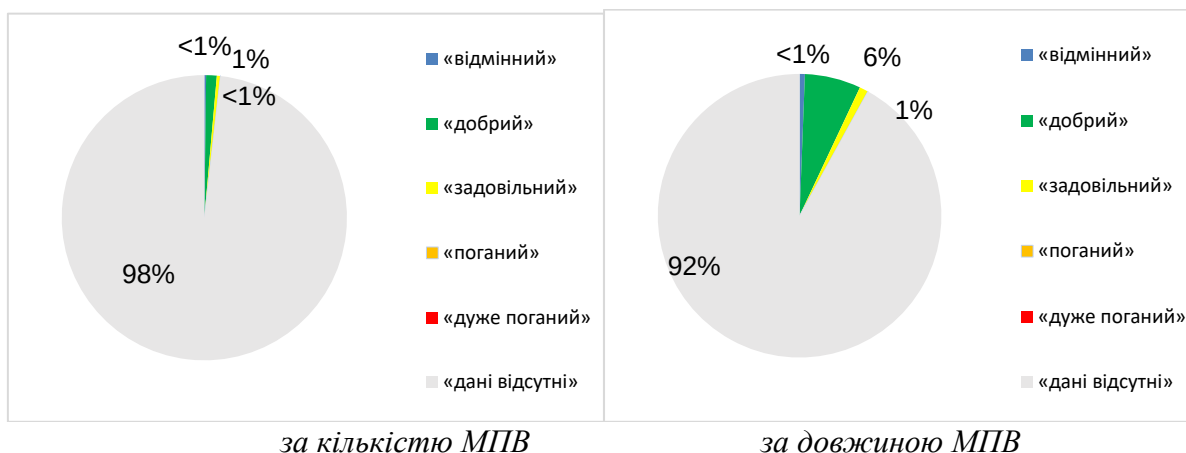
Рисунок 19. Оцінка екологічного стану лінійних МПВ РБР Південного Бугу
