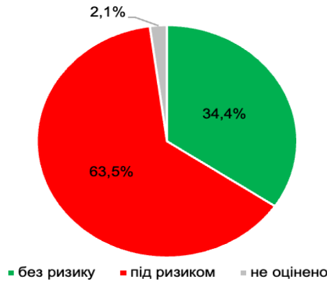
Рисунок 10. Оцінка ризику досягнення доброго екологічного стану / потенціалу за результатами оцінки антропогенних навантажень: гідроморфологічні зміни
