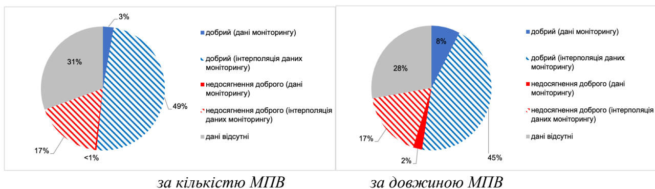
Рисунок 17. Оцінка хімічного стану лінійних МПВ РБР Південного Бугу
