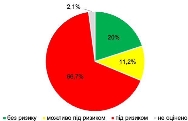
Рисунок 11. Узагальнена оцінка ризику досягнення доброго екологічного стану / потенціалу МПВ
