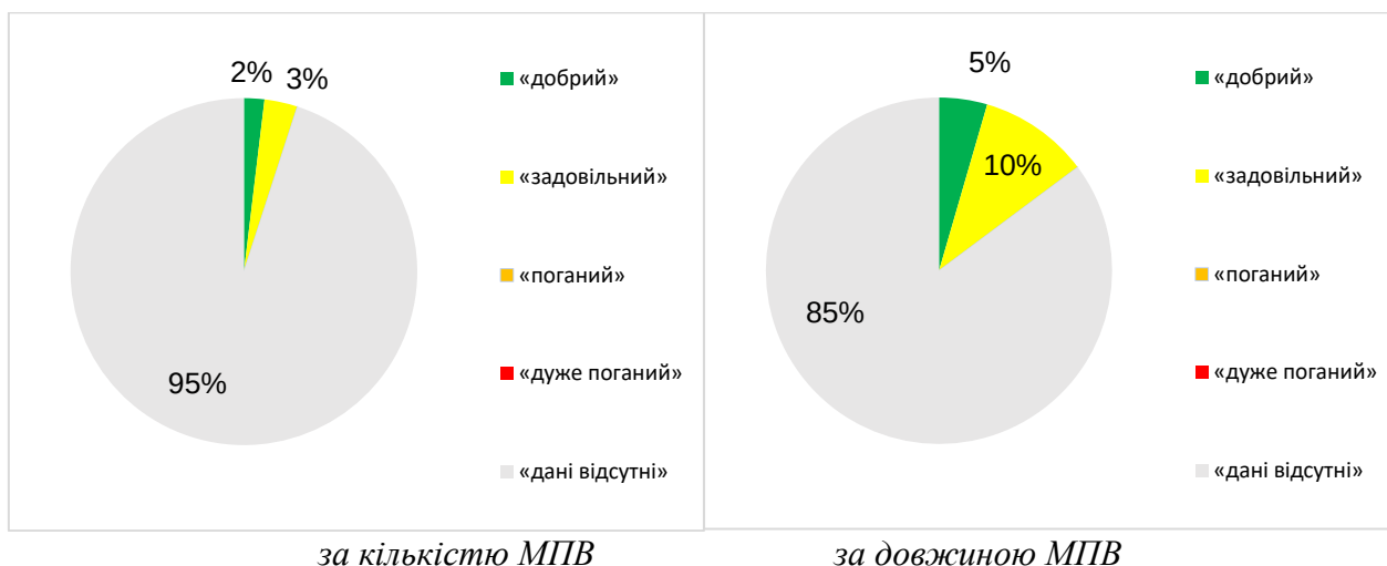
за кількістю МПВ за довжиною МПВ Рисунок 21. Оцінка екологічного потенціалу полігональних МПВ РБР Південного Бугу
