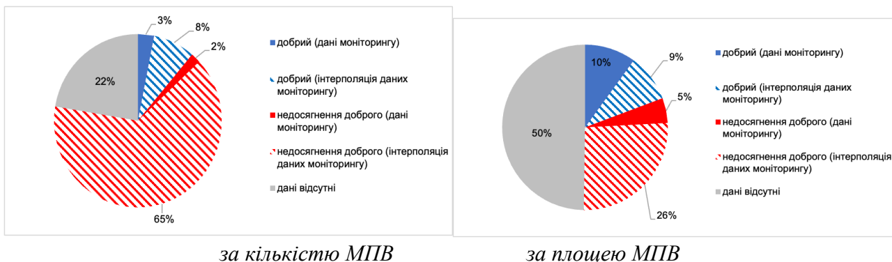
Рисунок 18. Оцінка хімічного стану полігональних МПВ РБР Південного Бугу
