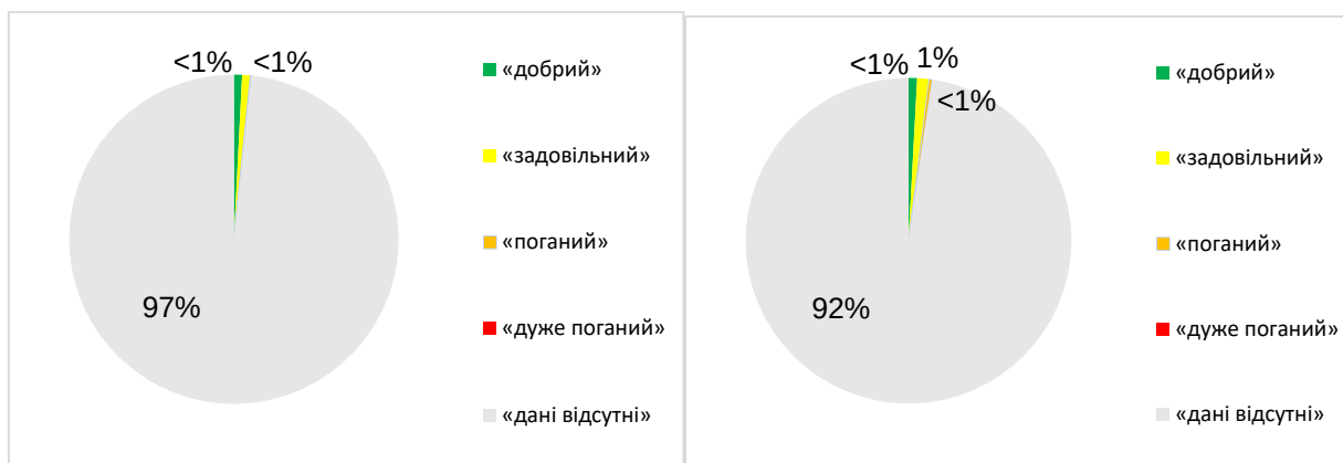
за кількістю МП за довжиною МПВ Рисунок 20. Оцінка екологічного потенціалу лінійних МПВ РБР Південного Бугу
